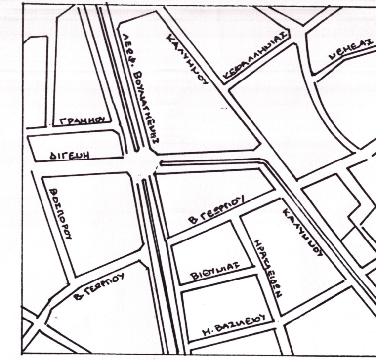
ΑΠΟΣΠΑΣΜΑ ΡΥΜΟΤΟΜΙΚΟΥ 1:5000
